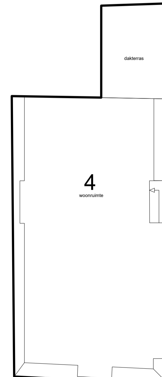
Zolderverdieping schaal 1:100
